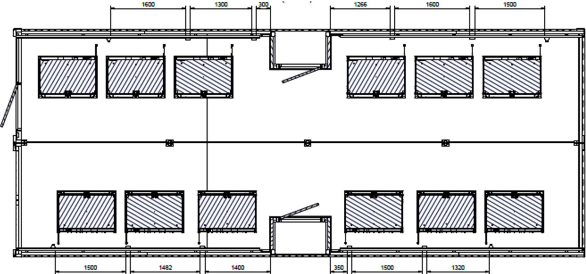
Section B-B (1 : 50)
