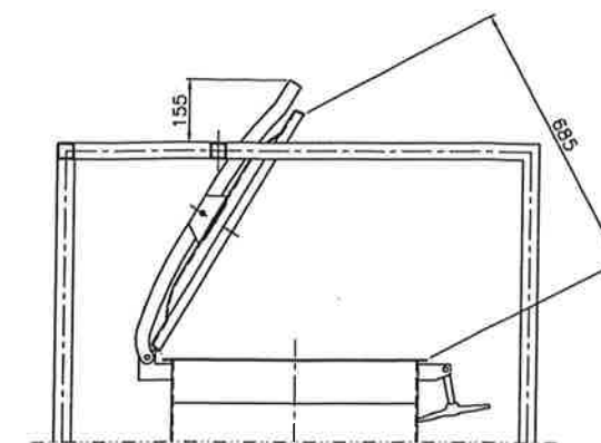
Detalje af åbning af låg på balancetank 300 L
