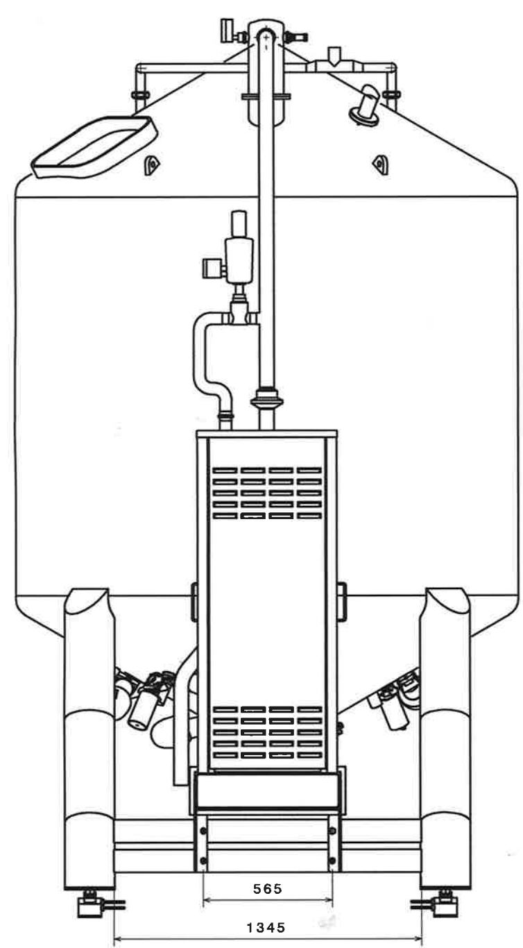
Right view Scale: 1:15
