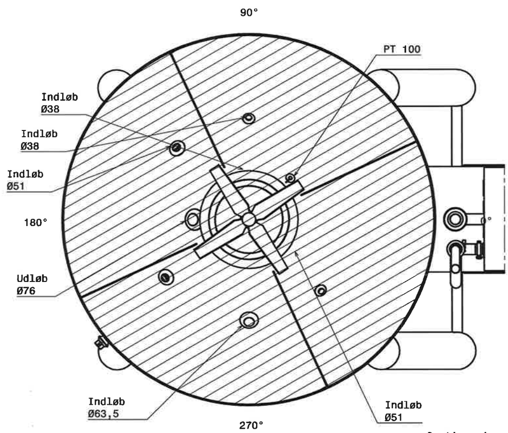
Section view A-A Scale: 1:15
