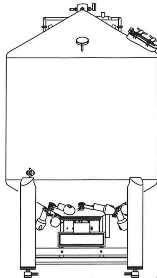
Left view Scale: 1:15
