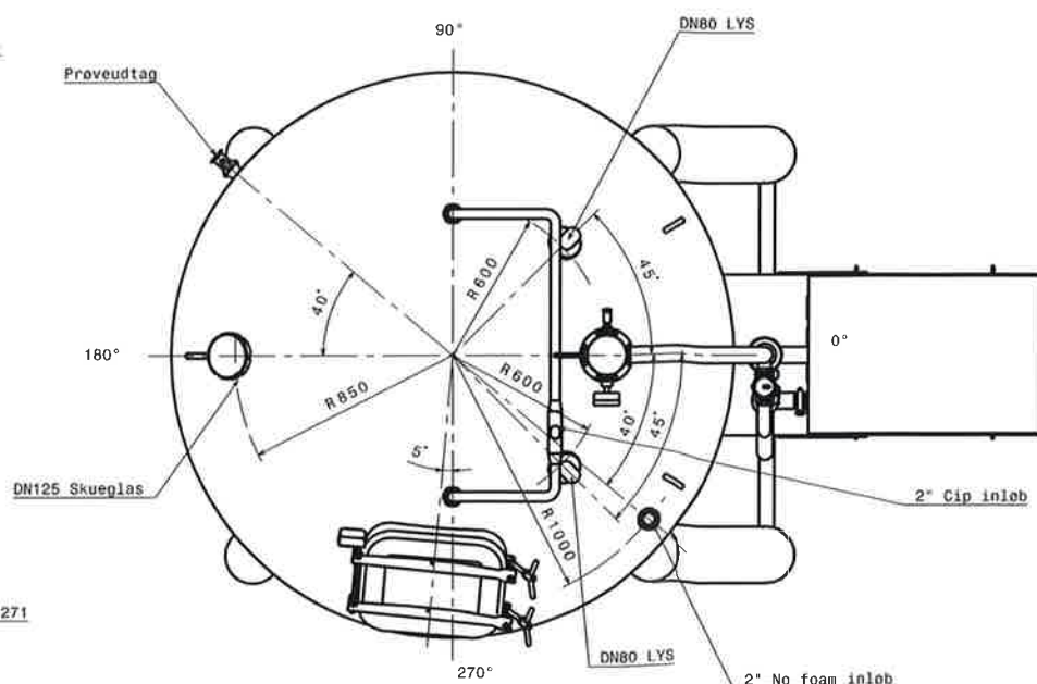
Top view Scale: 1:15
