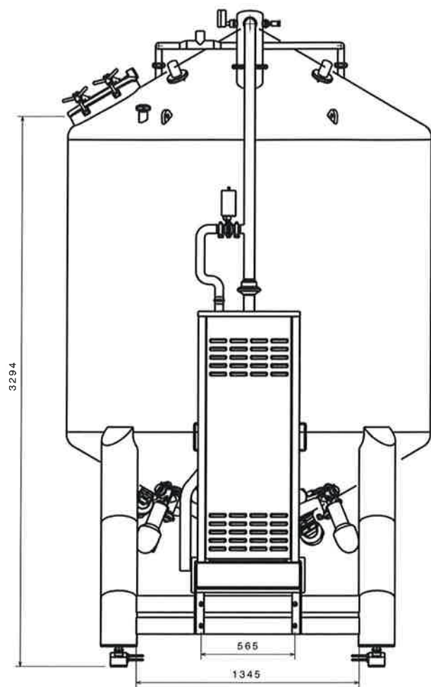
Right view Scale: 1:15
