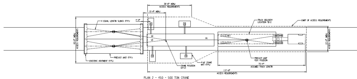
PLAN 2 - 450 - 500 TON CRANE
